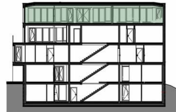
Schnitt
